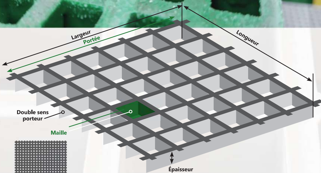
Portée (espace entre 2 plots fixes)
